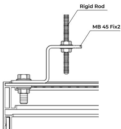
Pendant Rigid suspension
