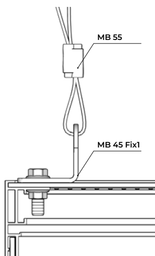
Flexible Wire pendant
